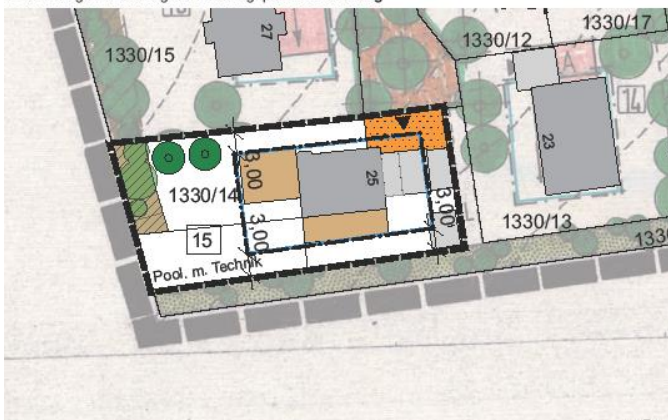
Darstellung rechtskräftiger Bebauungsplan n. Änderung
